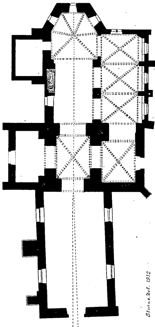
ÉGLISE D'ESQUERMES. — 1. Plan
