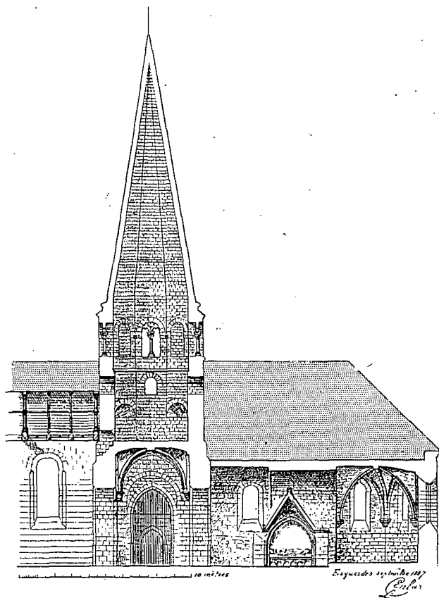
ÉGLISE D'ESQUERDES. — 3. Coupe du clocher et du sanctuaire.
